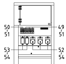
VIEW-D
